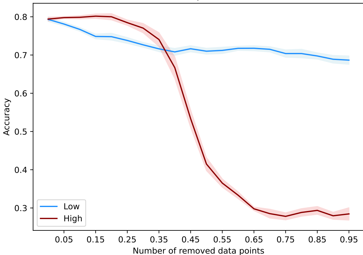
DataOob(1000, epochs=15) - adult
